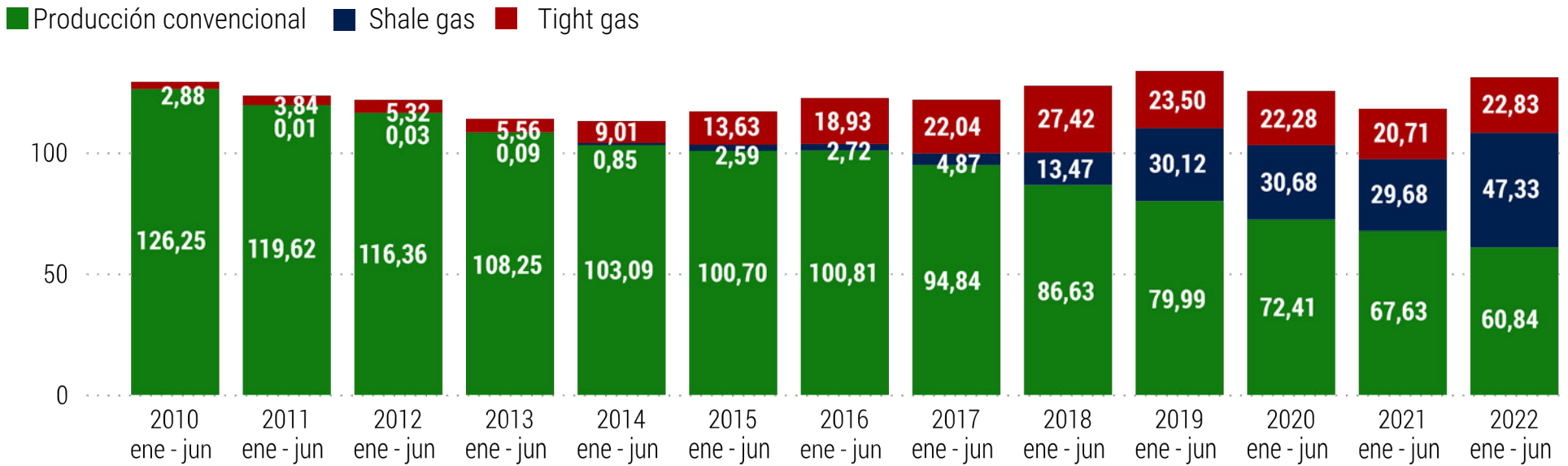
Producción bruta de gas por tipo de recurso en m³/día. Enero - junio 2010-2022
