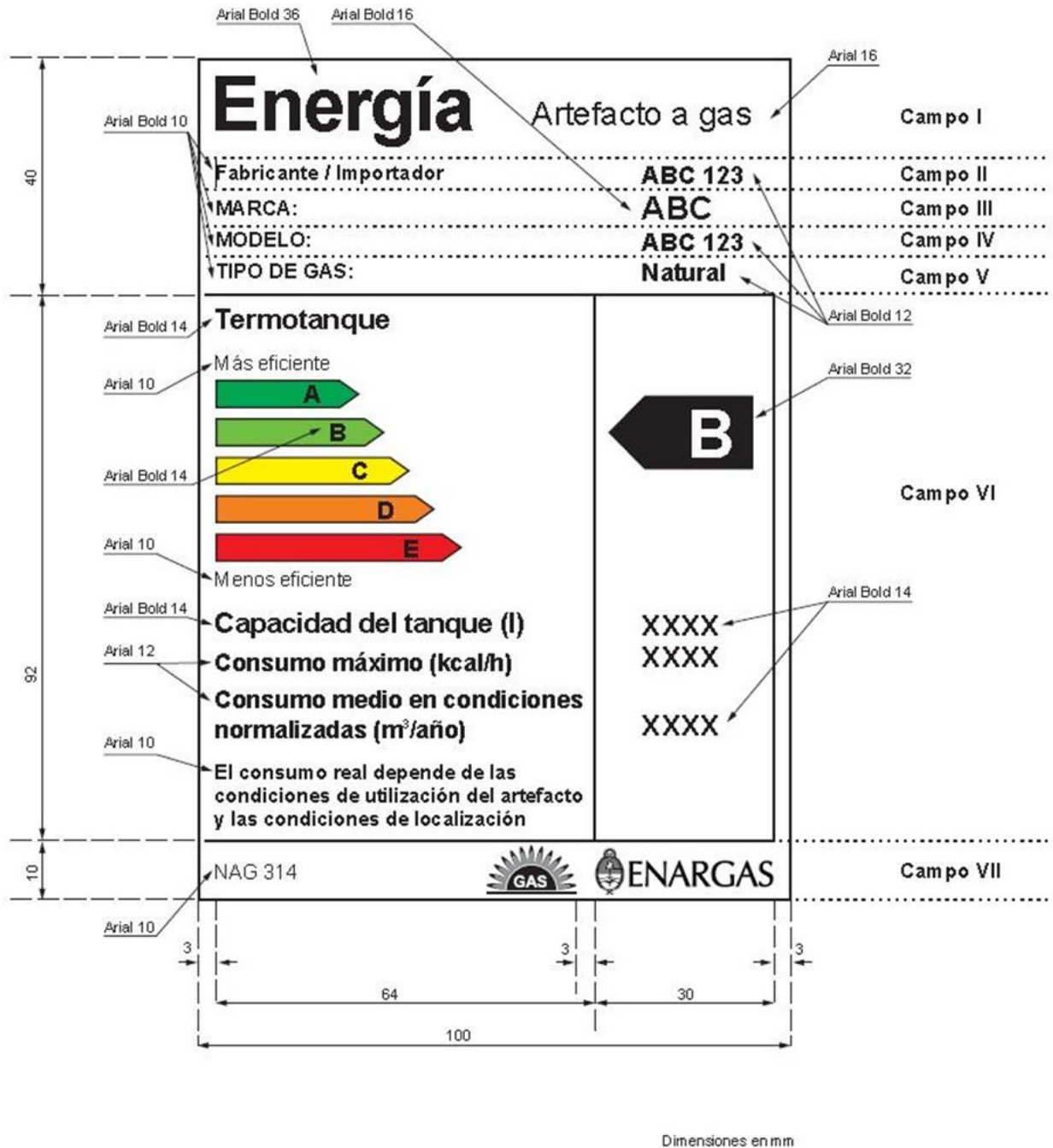
Figura E.1 - Etiqueta para aparatos de producción de agua caliente por acumulación (termostanques)
